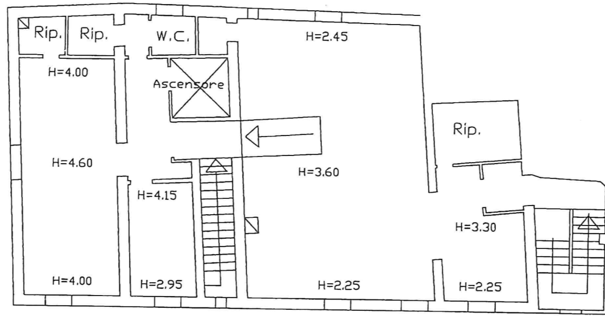
Piano Primo
